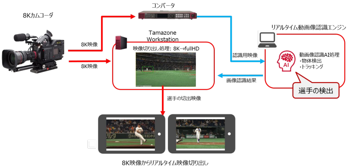
<8K 映像からのリアルタイム映像切り出し構成図>
