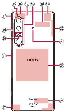
背面
