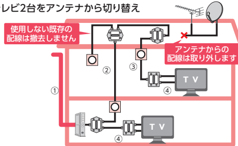
【例】テレビ2台をアンテナから切り替え
