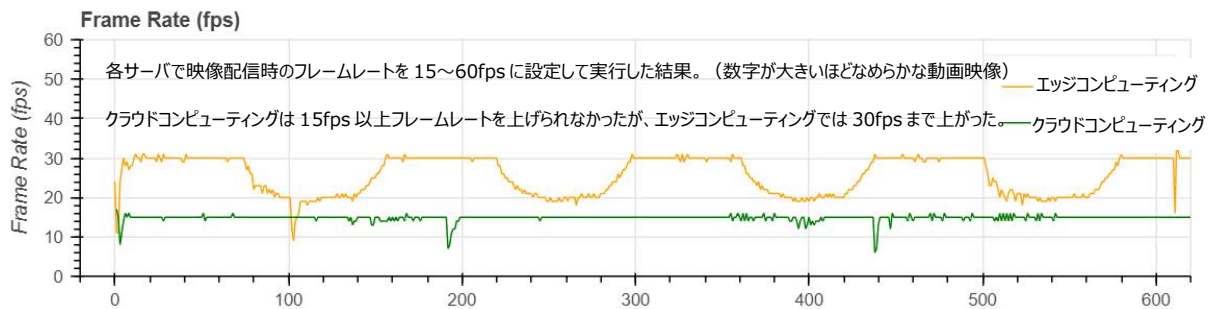
【測定例：クラウドレンダリングを一定時間実行した際のクライアントにおけるフレームレート】
