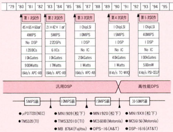
図16 高効率音声符号化の技術的進展 Figure 16 Progress of high efficiency voice CODEC
