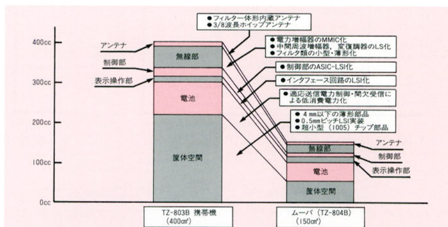
図8 150cc化のための主要技術 Figure 8 Technologies for 150cc Portable Radio Telephone Unit
