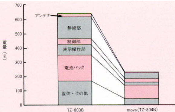
図9 超小型携帯機—mova—の重量配分
