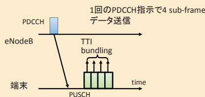
図8 TTI bundling
