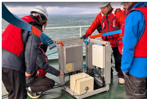
基地局装置設営
